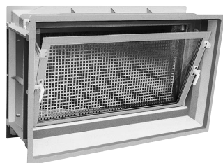
Okno z ościeżnicą typu Z skrzydło uchylne (na zdjęciu także kratka ochronna)
