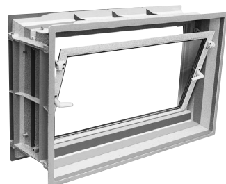
Okno z ościeżnicą typu Z, skrzydło uchylne (bez kraty ochronnej)
