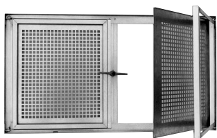
Okno typu SD2 dwuskrzydłowe, otwieralna kratka i skrzydło szklone z możliwością demontażu. Słupki oporowe przytwierdzone do ramy
