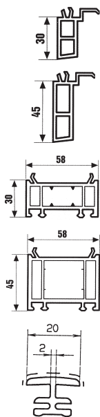
Okno typu MDK z przyłączem na suszarkę do prania
