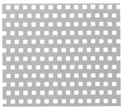
Otwory kwadratowe w układzie mijanym
